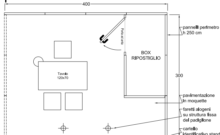
pianta stand 4x3
